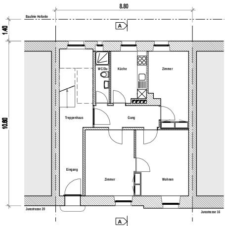
Erdgeschoss bestehend
