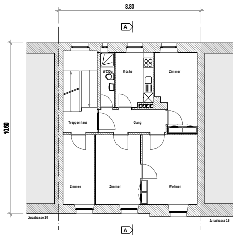
Obergeschoss 4 bestehend
