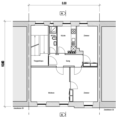
Obergeschoss 1 bis 3 bestehend
