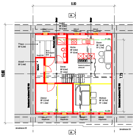
Dachgeschoss Ausbau neu
