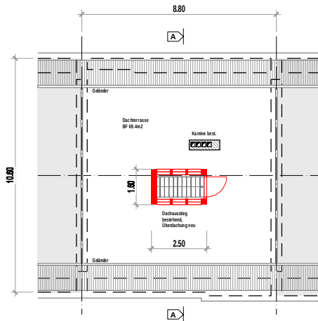
Dachaufsicht bestehendneu
